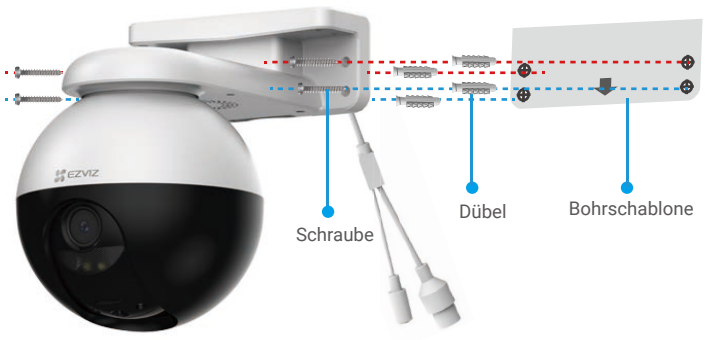
Abb. 2 Wandmontage
